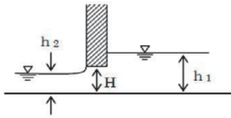
圖7-3-3 水門的逕流型態與各項要素
